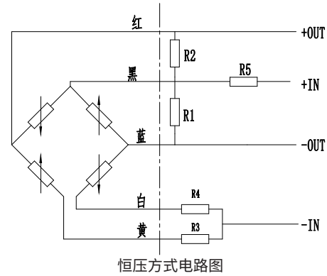
恒压方式电路图
