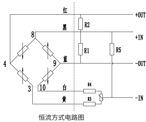
恒流方式电路图
